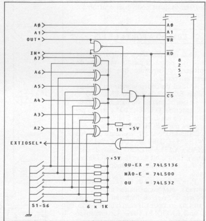
Figura 6 - Seleção por portas (programável)
